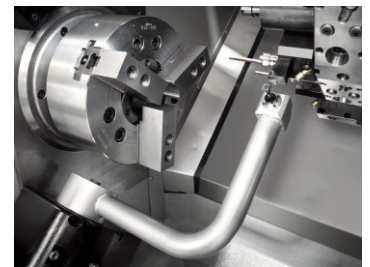
Tool setter
